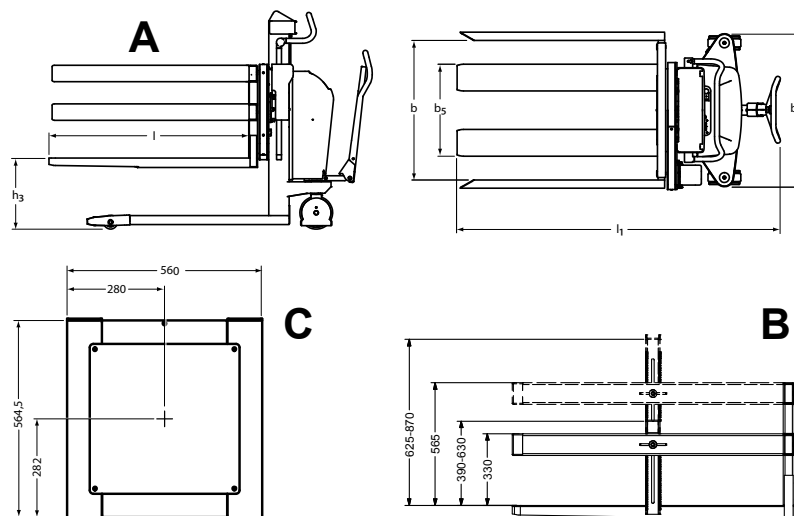
A: Rotator med dubbla sidostöd.
