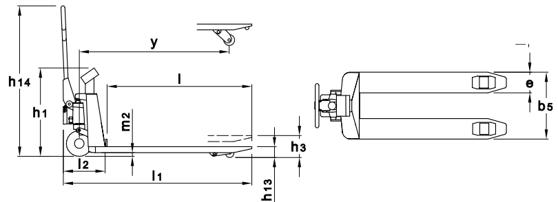
BFC6 transporterar och väger i en och samma arbetscykel.
