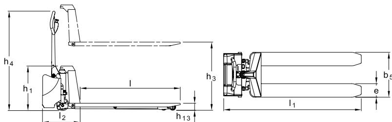
Mycket låg pumpkraft är kännetecknande för HL 1005, som är försedd med fotskydd och neutralställning av handtaget.
